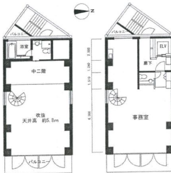
《5階平面図》
