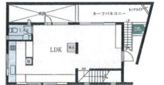
2F 48.51㎡
